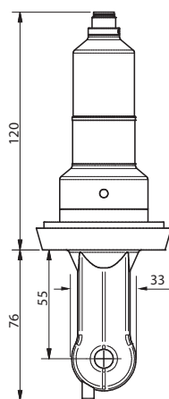
Dairy pipe DN 50 SE680(N/X)-C1N4U00M
