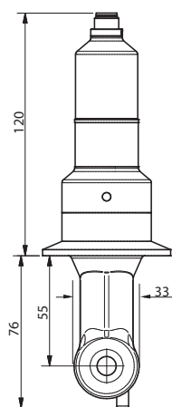
Clamp 2" SE680(N/X)-J2N4U00M
